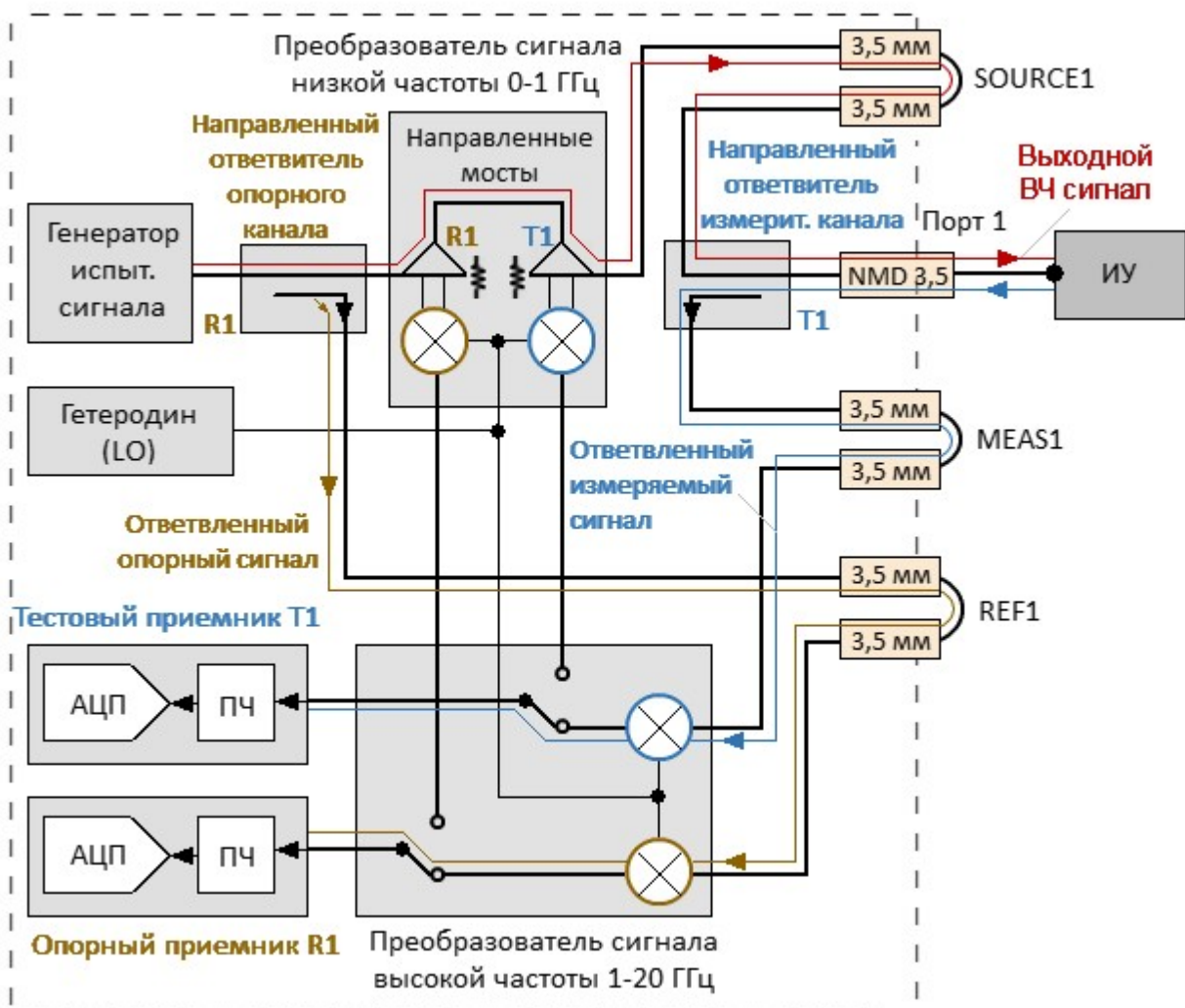
Рисунок – Анализатор С2420, распространение сигнала в общем режиме (диапазон от 1 до 20 ГГц)
