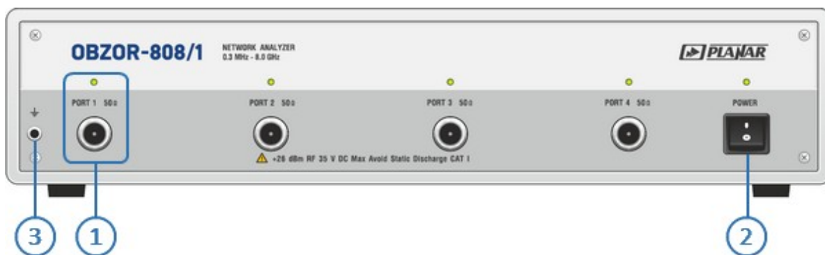
Рисунок – Передняя панель ОБЗОР-808/1
