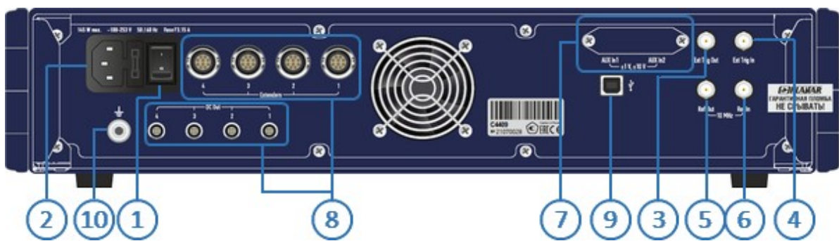
Рисунок – Задняя панель S4409
