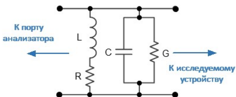
Рисунок – Предустановленная согласующая цепь
