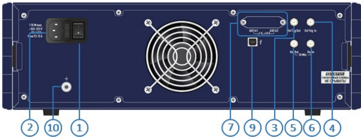
Рисунок – Задняя панель S1420, S2420
