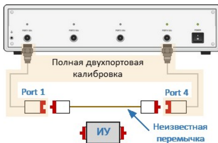
Рисунок – Второй этап калибровки с неизвестной перемычкой SOLR
