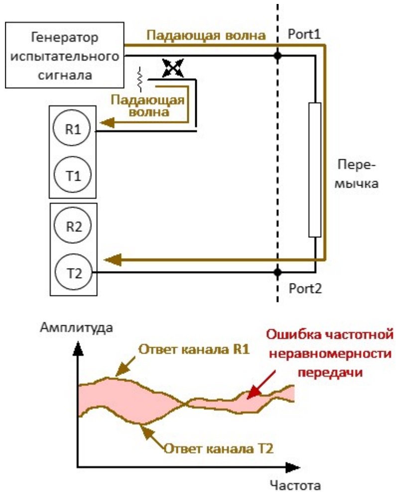
Рисунок – Ошибка частотной неравномерности передачи
