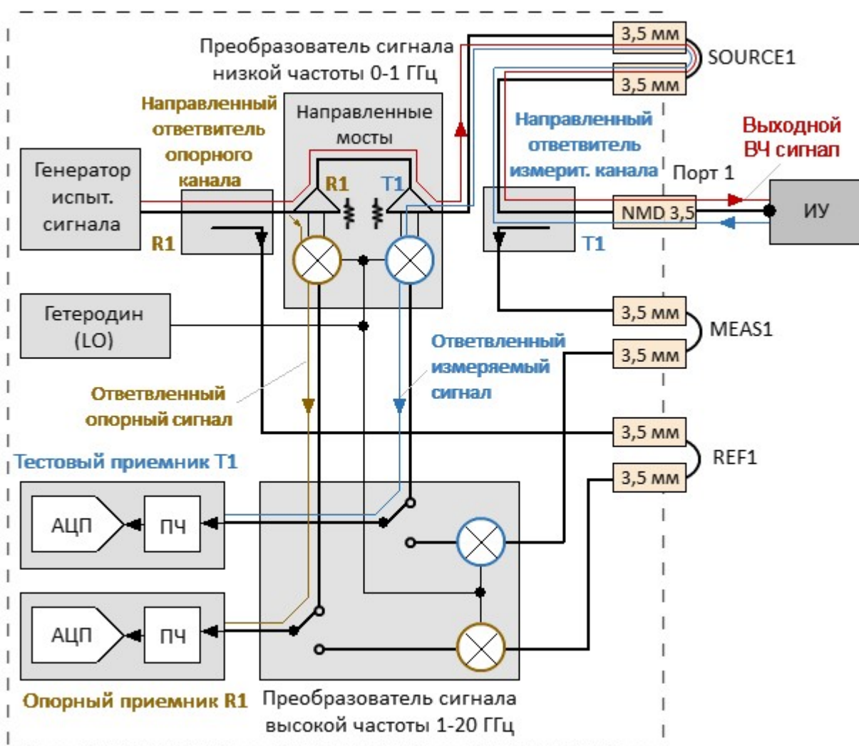
Рисунок – Анализатор С2420, распространение сигнала в общем режиме (диапазон от 100 кГц до 1 ГГц)
