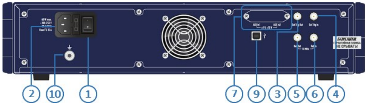
Рисунок – Задняя панель S1409, S2409
