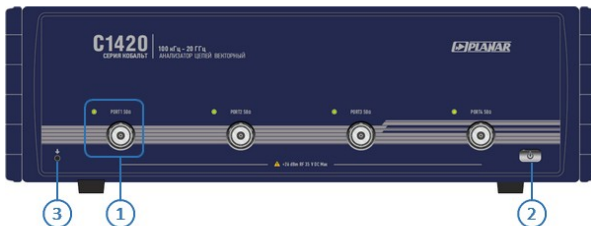
Рисунок – Передняя панель C1420
