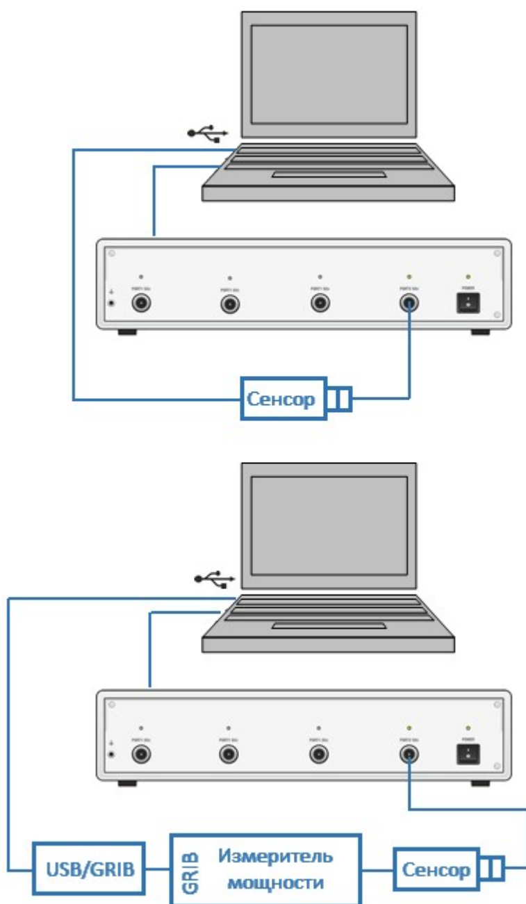
Рисунок – Пример подключения измерителя мощности
