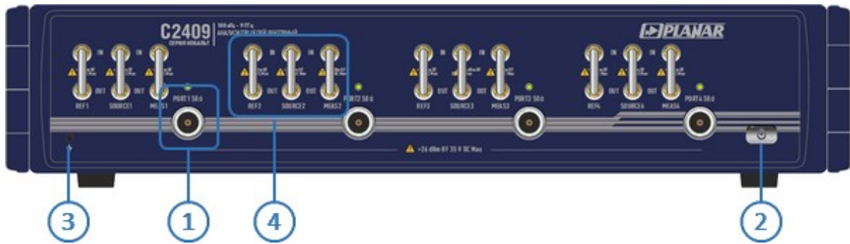
Рисунок – Передняя панель C2409
