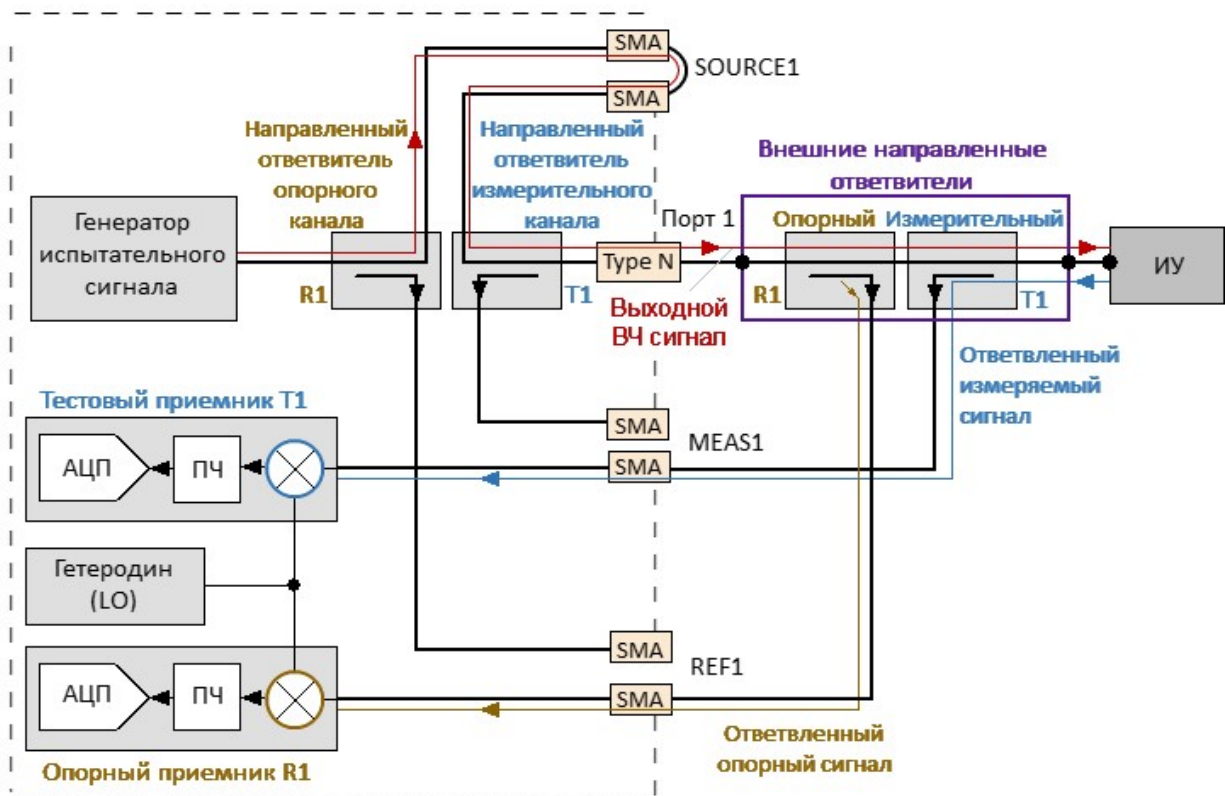
Рисунок – Анализатор C2409, распространение сигнала в режиме прямого доступа
