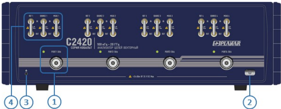
Рисунок – Передняя панель C2420
