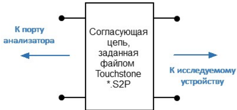
Рисунок – Пользовательская согласующая цепь
