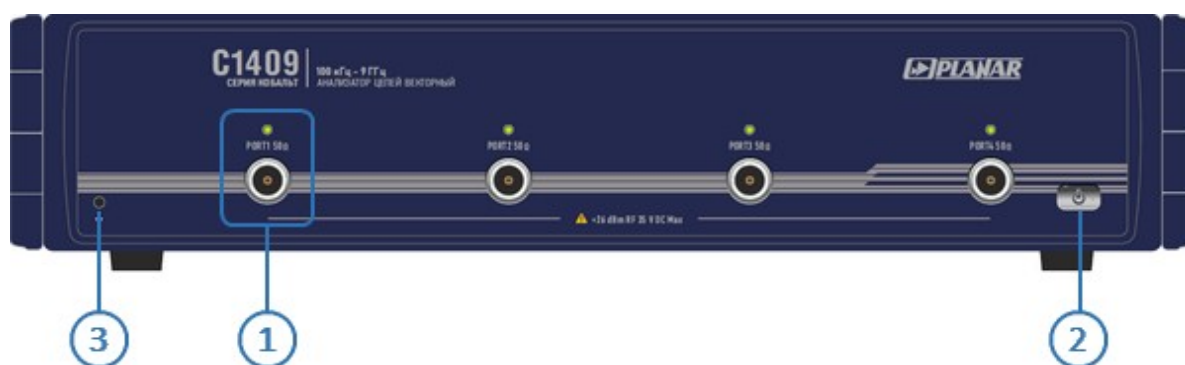
Рисунок – Передняя панель C1409
