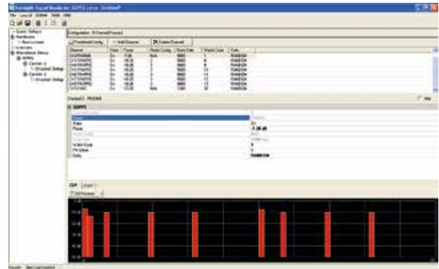
Интерфейс пользователя ПО PathWave Signal Generation для сигналов cdma2000, показывающий конфигурацию с несколькими несущими.
