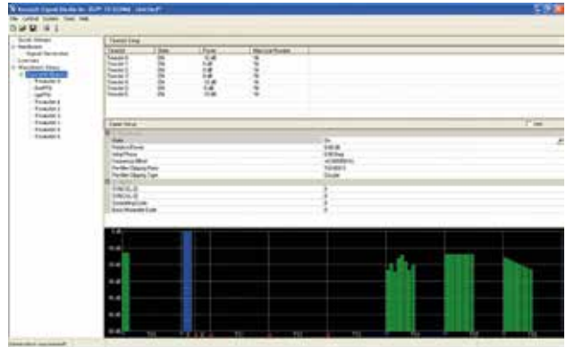
Интерфейс пользователя PathWave Signal Generation для сигналов TD-SCDMA, показывающий конфигурацию сигнала нисходящего канала с 6 несущими.
