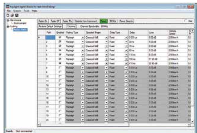
Интерфейс пользователя программы PathWave Signal Generation для имитации замираний сигналов в реальном времени (N7605C).
