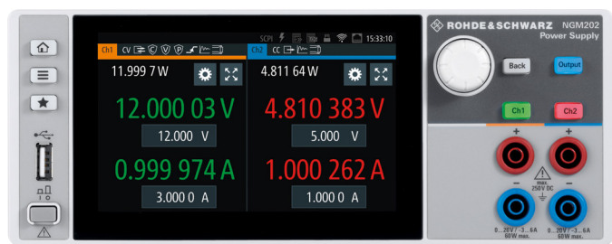
R&S®NGM202, вид спереди
