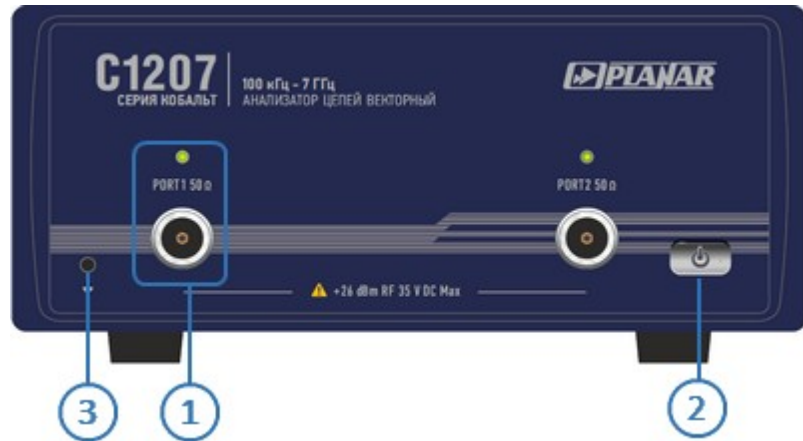
Рисунок 14– Передняя панель
