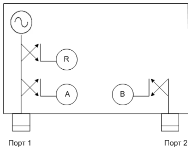
Рисунок 4.3 Структурная схема анализатора
