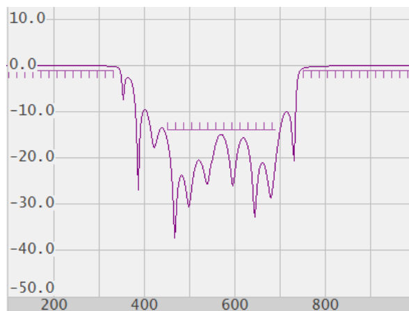
Рисунок 6.15 Линия шаблонов
