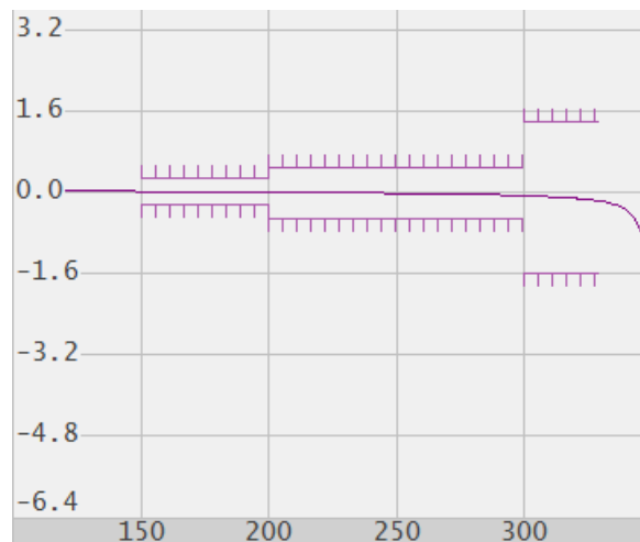
Рисунок 6.17 Пределы пульсаций
