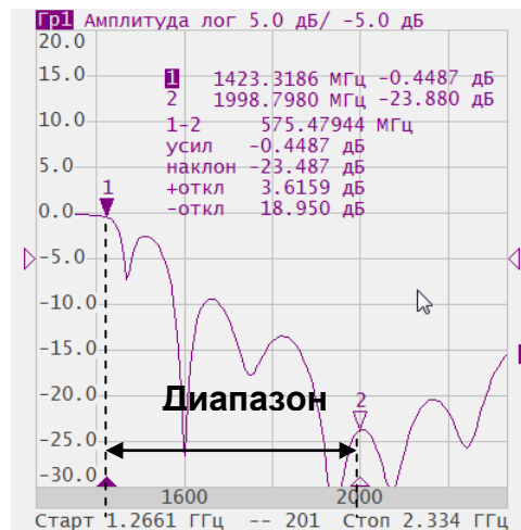
Рисунок 6.10 Функция неравномерности.
