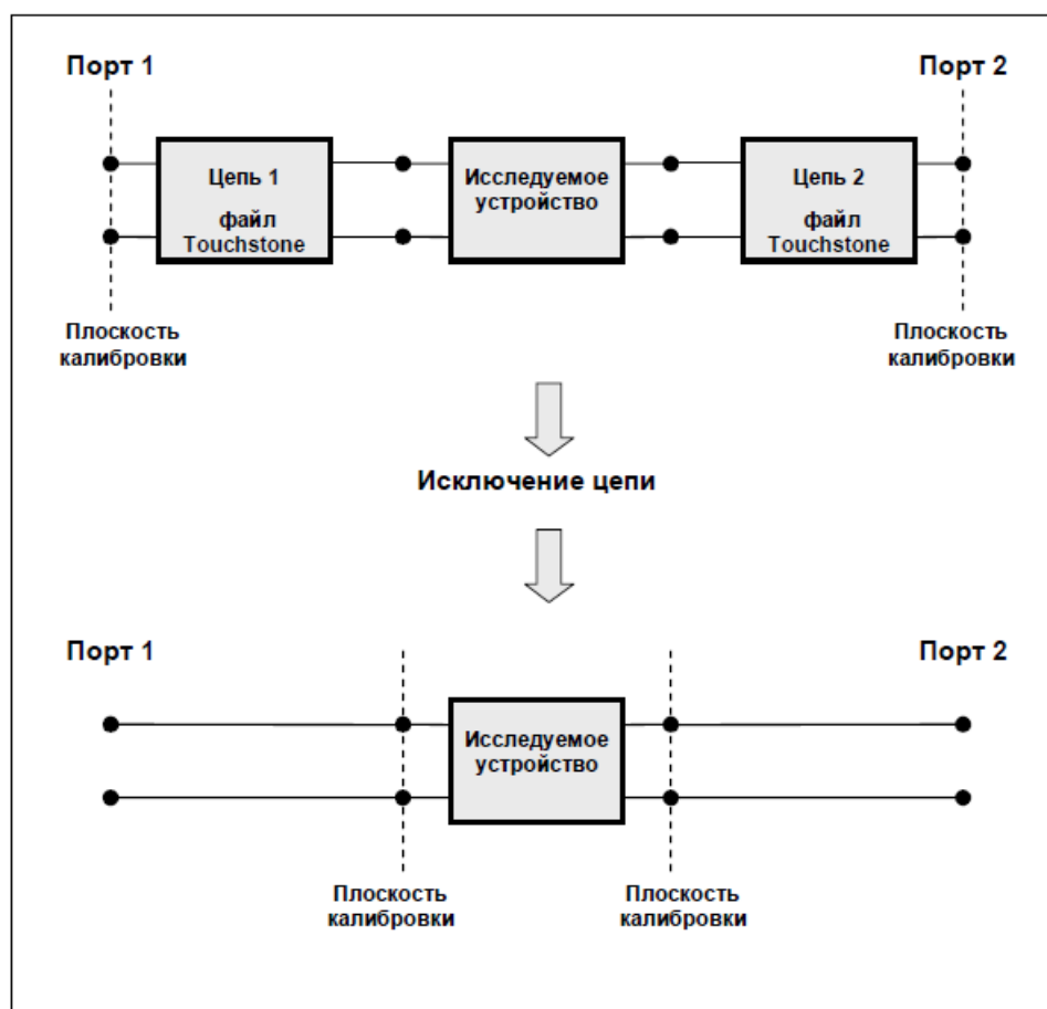
Рисунок 6.13 Исключение цепи
