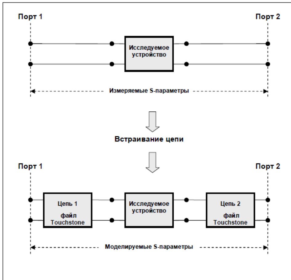
Рисунок 6.14 Встраивание цепи
