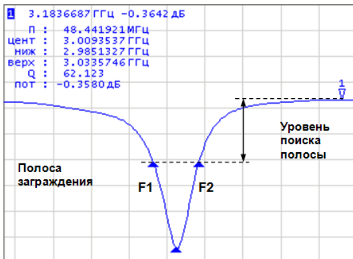
Рисунок 6.9 Поиск полосы.
