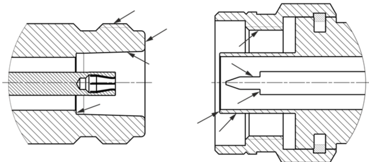
Рисунок 2 – Соединители тип N и III (розетка и вилка)
