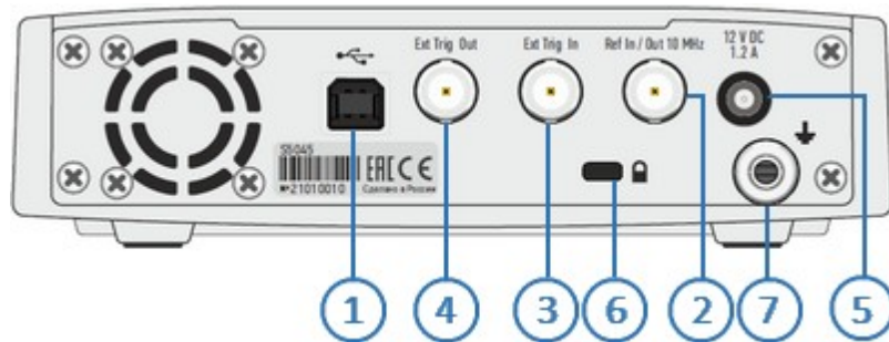
Рисунок 15 – Задняя панель
