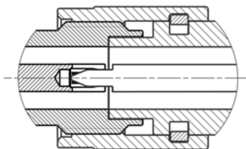
Рисунок 7 – Соединители тип 2,4 мм, 3,5 мм и IX(розетка слева, вилка справа)
