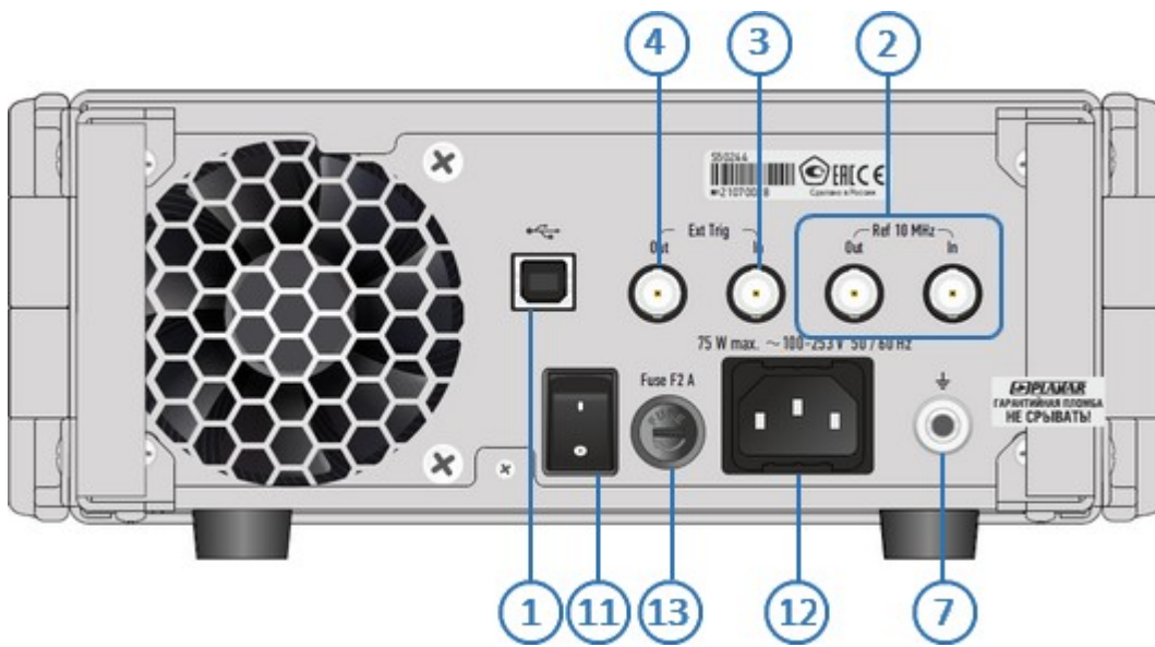
Рисунок 21 – Задняя панель
