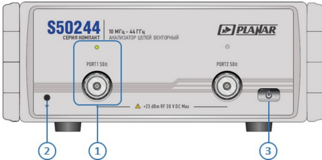
Рисунок 20 – Передняя панель
