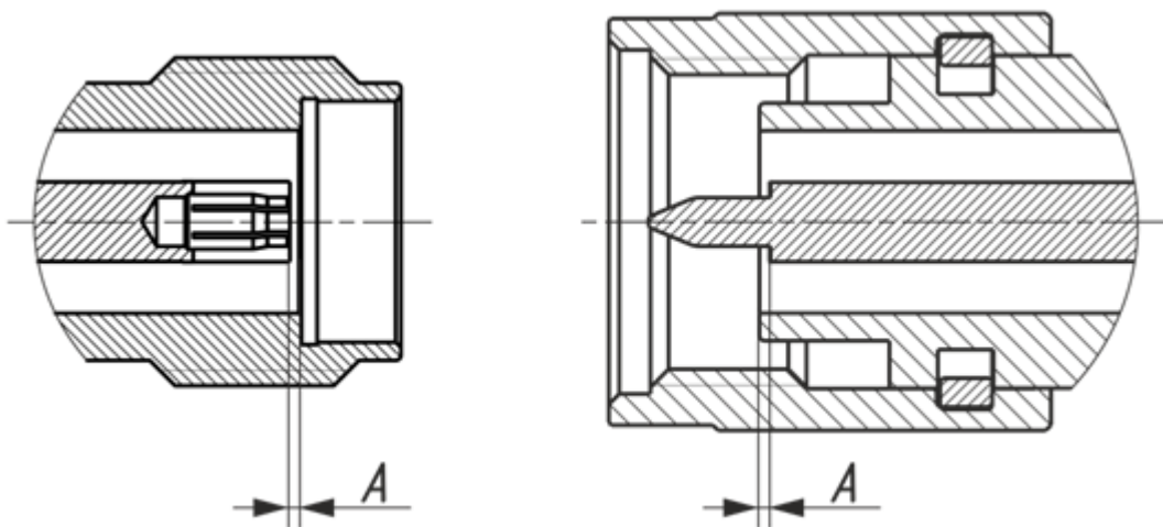
Рисунок 5 – Соединители тип 2,4 мм, 3,5 мм и IX (розетка и вилка)
