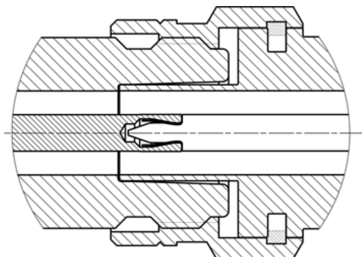
Рисунок 6 – Соединители тип N и III (розетка слева, вилка справа)
