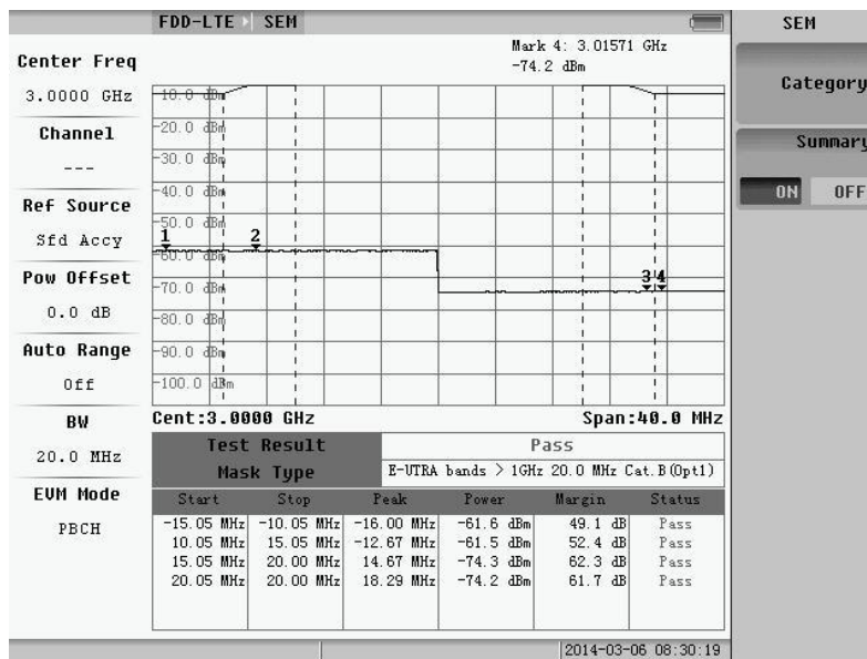
Fig.5.66 SEM menu
