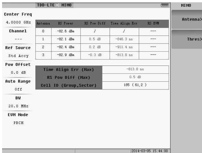
Fig.5.37 MIMO menu
