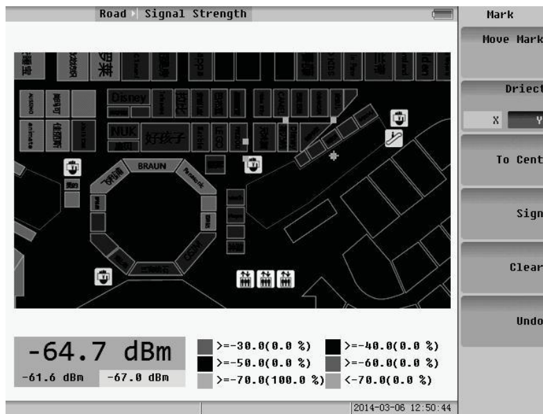
Fig.6.12 Sign free
