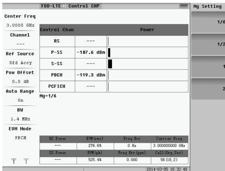
Fig.5.54 Ng submenu
