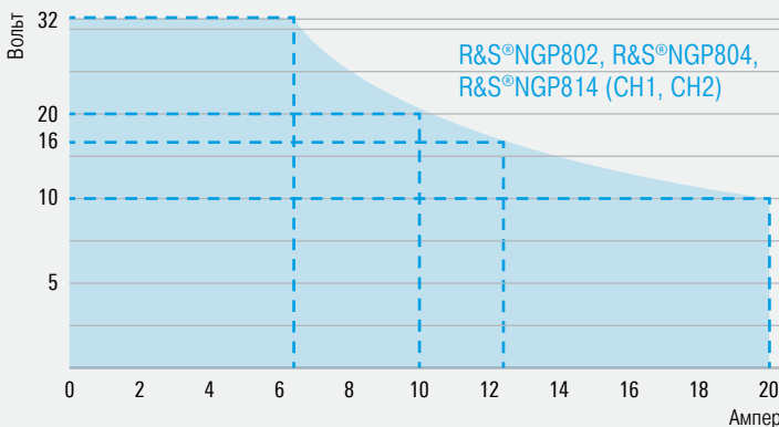
Функция FlexPower 32 В/20 А (макс. 200 Вт на канал)
