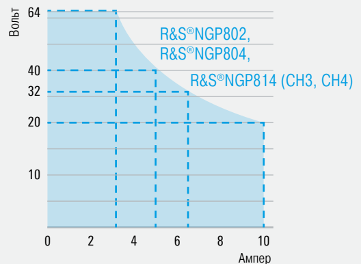
Функция FlexPower 64 В/10 А (макс. 200 Вт на канал)
